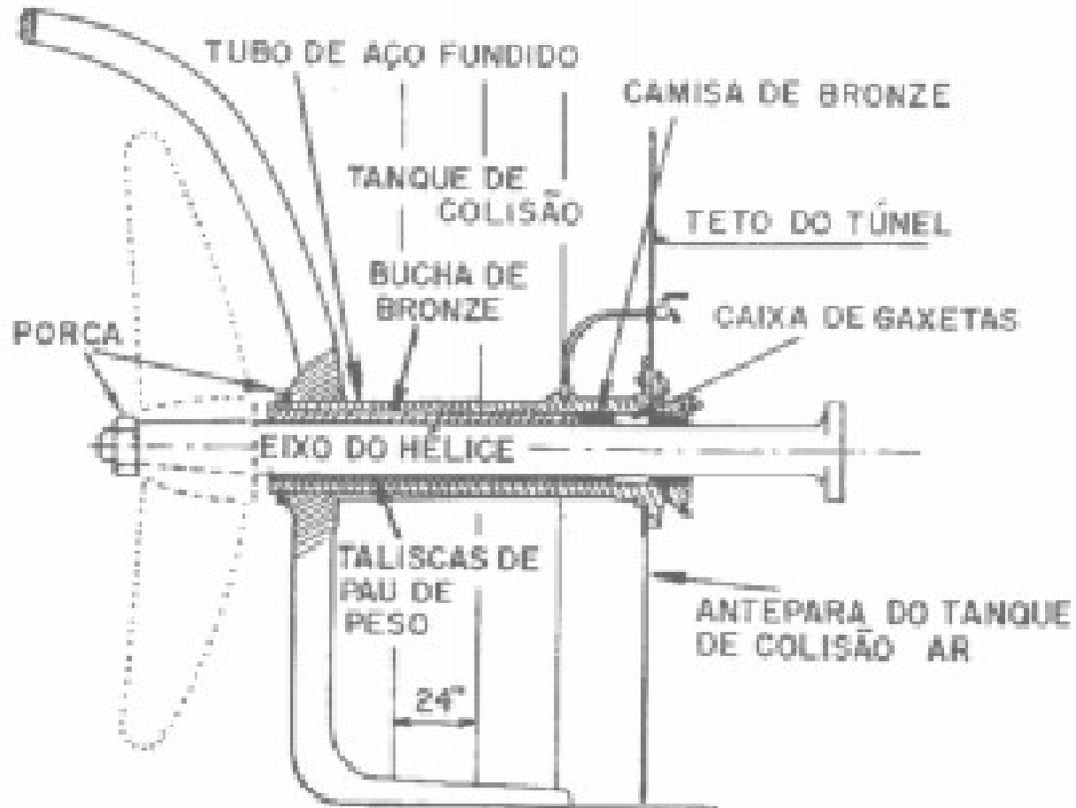
A - TUBO CURTO (1 MANCAL)
